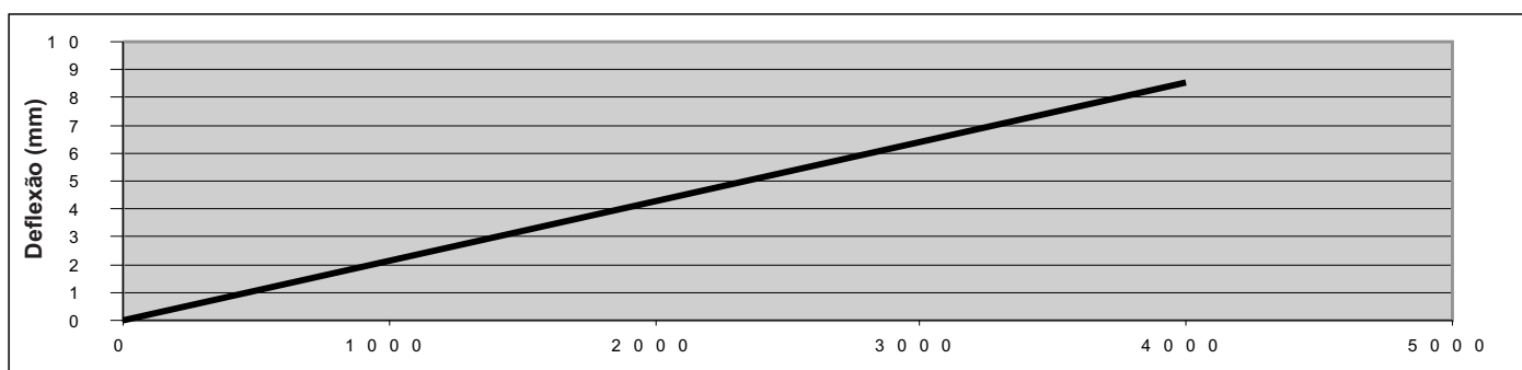
Curva "Carga x Deflexão"
